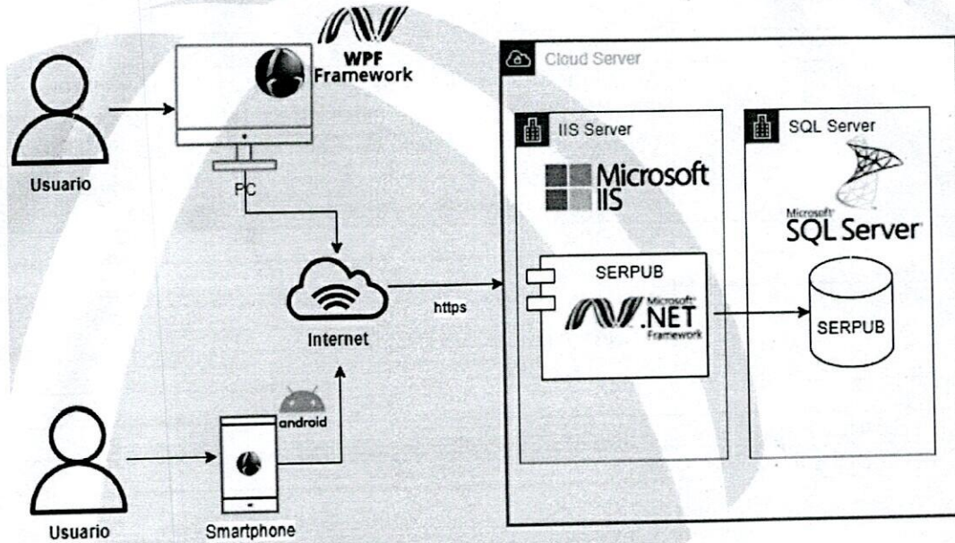
Ilustración 1 Arquitectura técnica de la infraestructura
