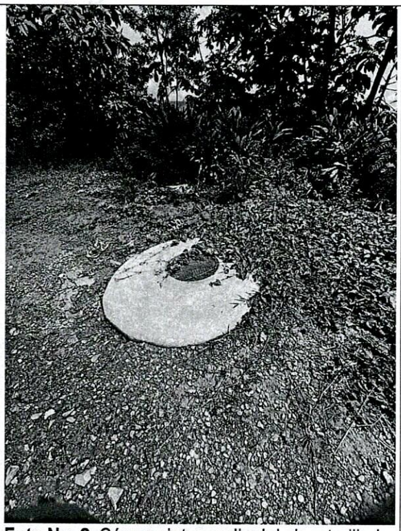
Foto No. 2. Cámara intermedia del alcantarillado La Gaviota.
