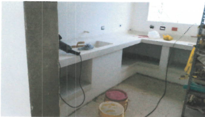
Se elabora la instalación del granito con relación de grano natural N°2, marmolina y cemento blanco.
