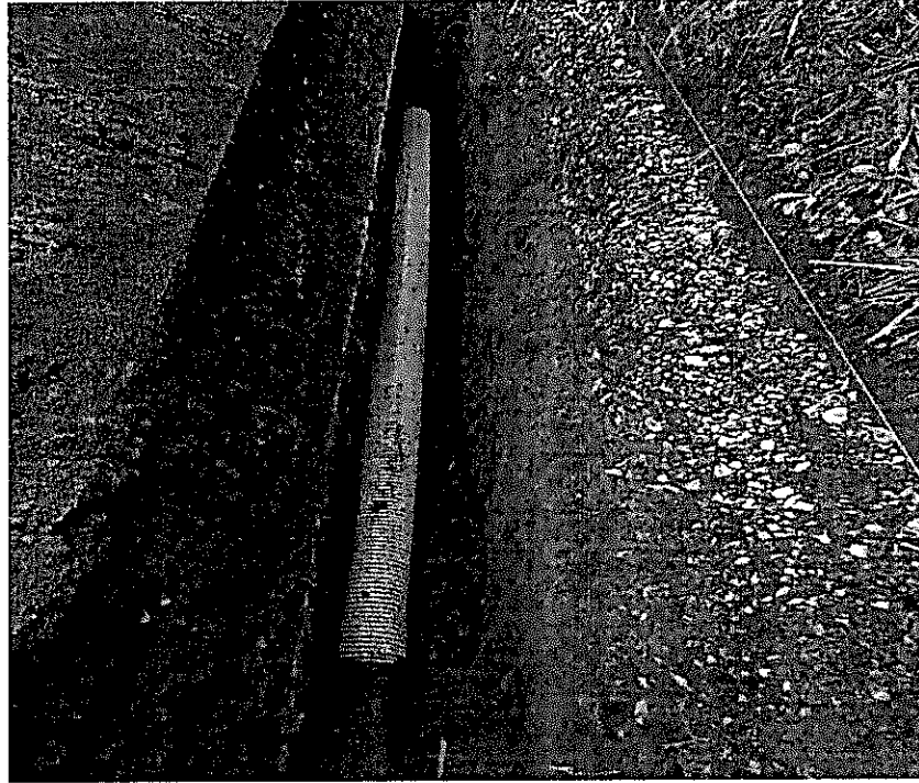
Instalación de tubería principal de 10" incluye cama en arena
