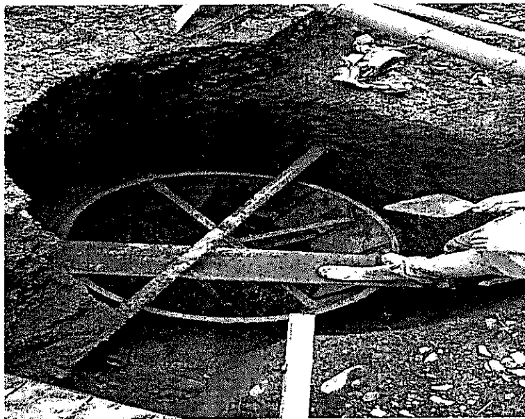
Vaciado de cámaras
