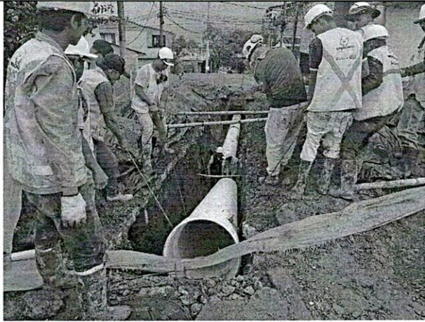
Instalación tubería
