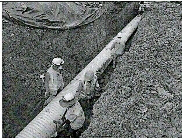
Instalación tubería
