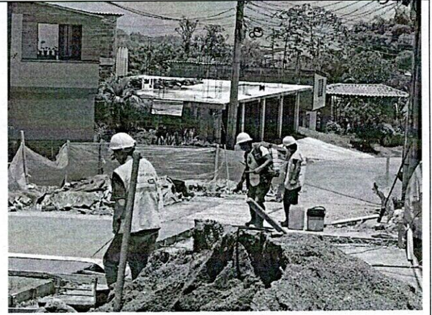
Vaciado de Concreto
