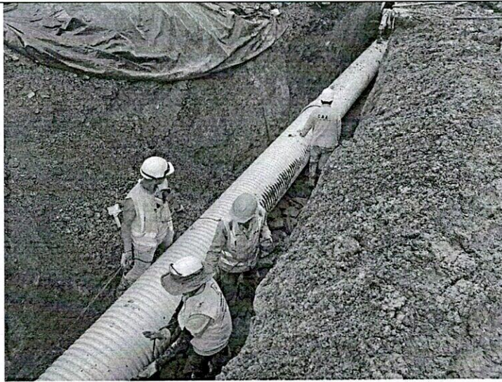
Instalación tubería
