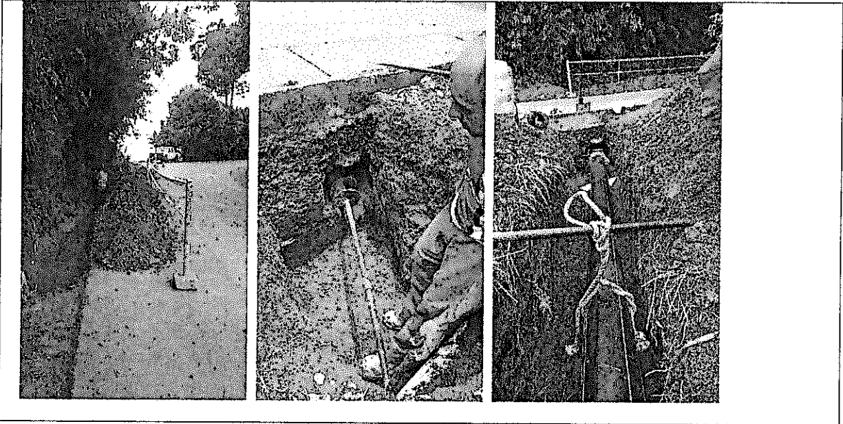
Proceso de perforación para atravesar la vía
