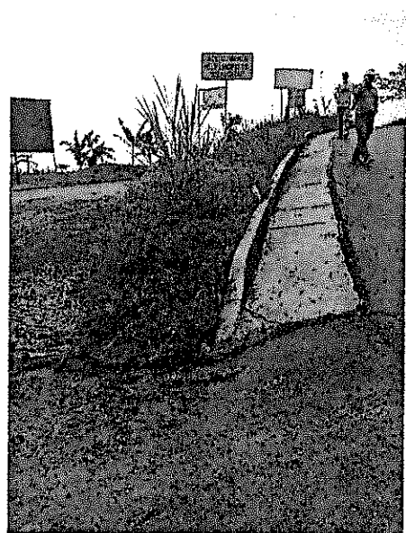
DAÑO DE TUBERÍA DE POLIETILENO EN EL SECTOR DE LA YEE
