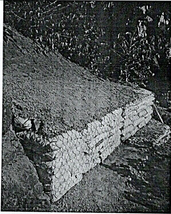
FOTO 3. Muro de gaviones con sacos rellenos de suelo cemento 10:1
