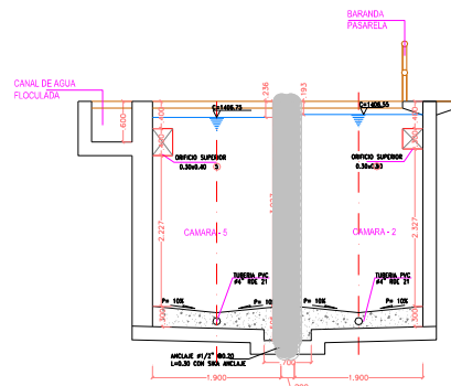
CORTE D-D'
