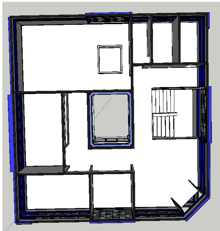
Planta general segundo piso zona administrativa.
