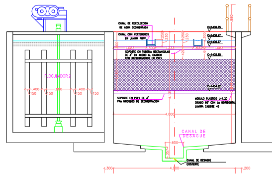
CORTE F-F'
