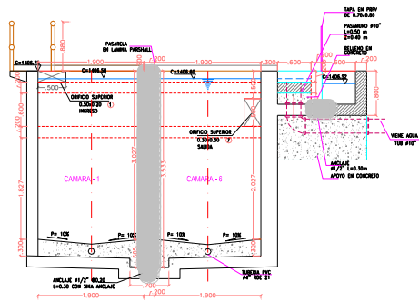
CORTE E-E'
