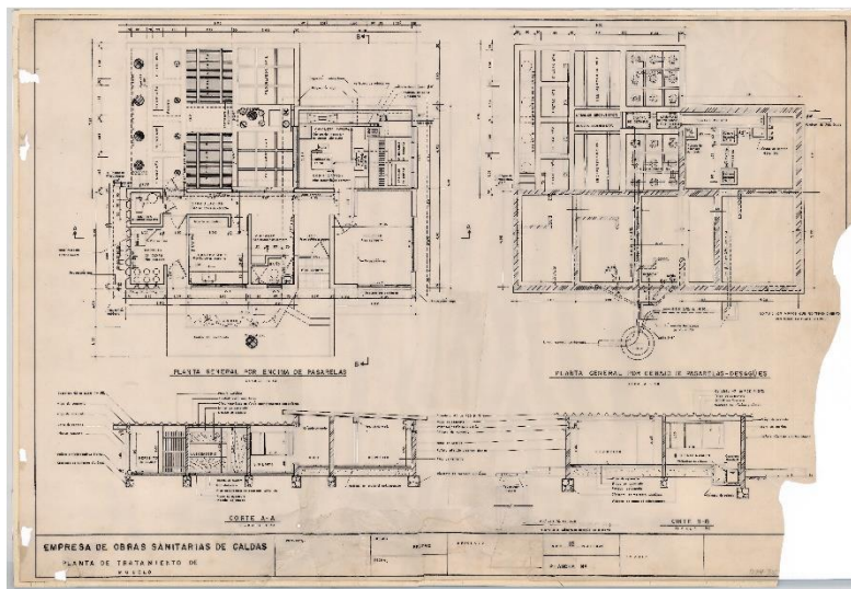
Planos originales realizado a mano de la planta de Neira. Empocaldas.
