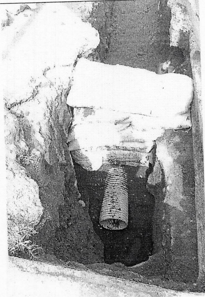
Imagen 11. Instalación tubería PVC corrugada de 14".
