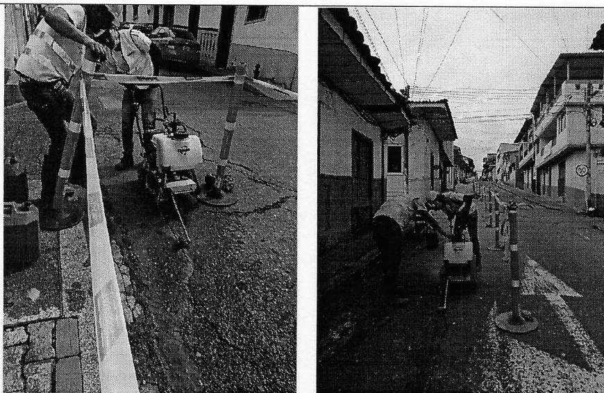
Imagen 2. Corte con disco abrasivo.
