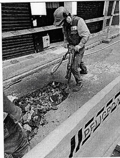
Imagen 5. Demolición de estructuras en concreto hidráulico y asfáltico con compresor con martillo.
