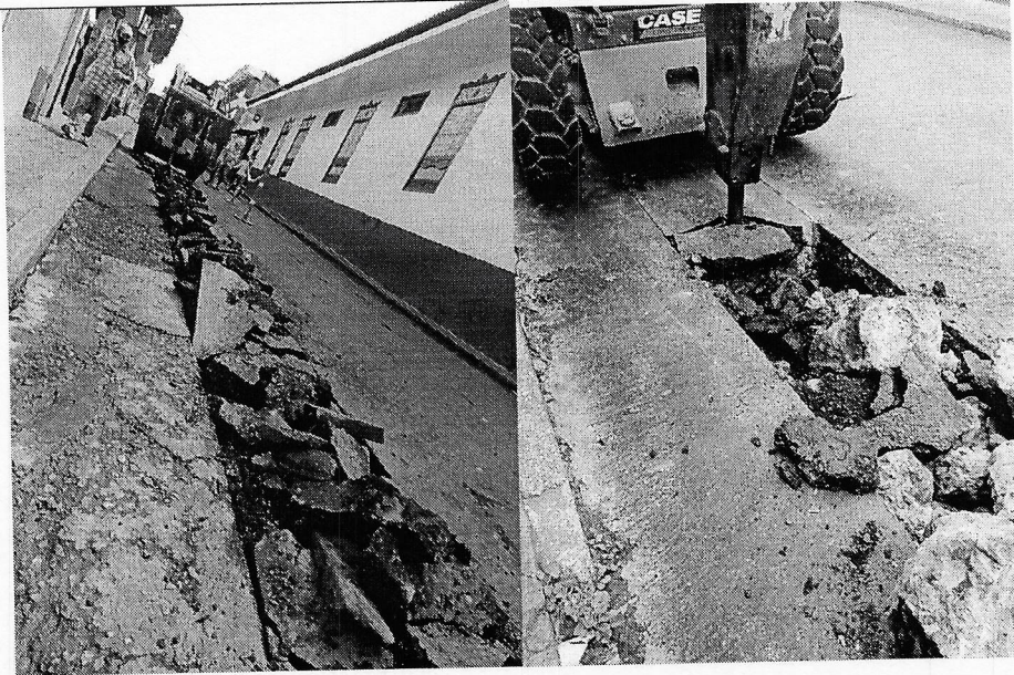
Imagen 4. Demolición de estructuras en concreto hidráulico y asfáltico con mini cargador con martillo.
