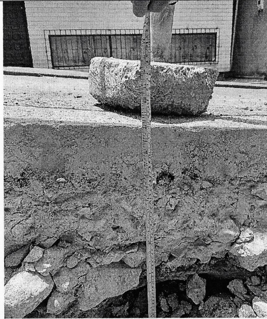
Imagen 6. Espesor pavimento existente.
