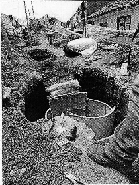
Imagen 13. Formaleta para construcción de cámara.
