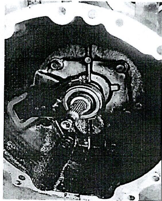
Cambio retenedor cigüeñal y empaque cárter
