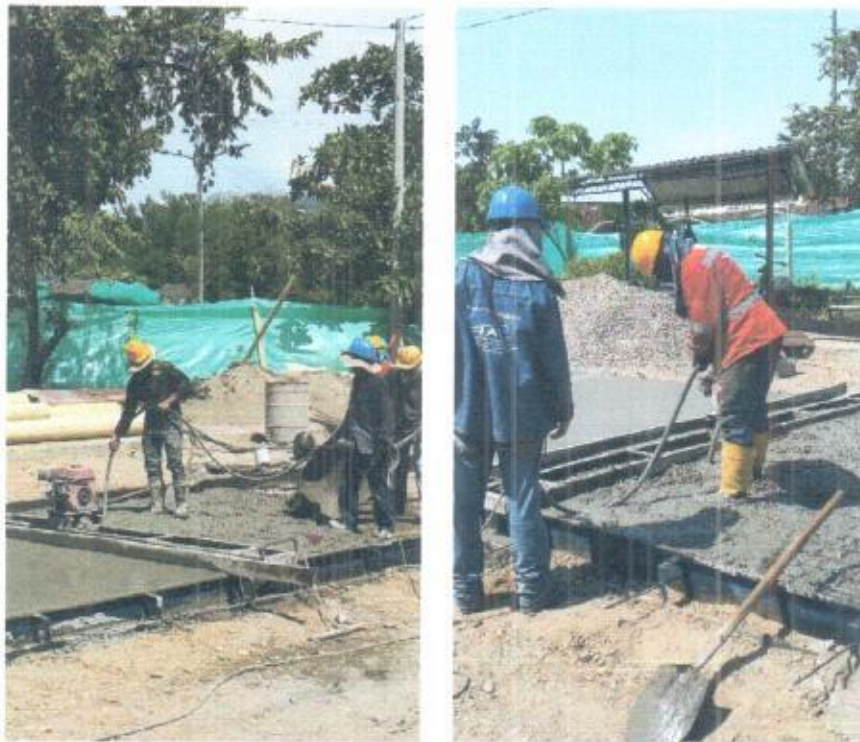
Foto 17 Y 18. Vibrado de la mezcla del pavimento de concreto.
