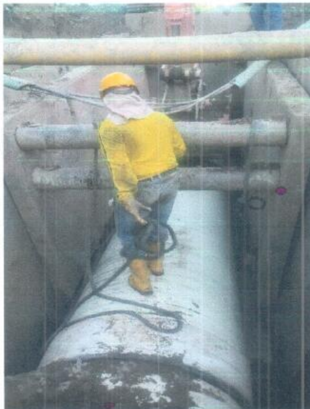
Foto 1. Instalación de tubería de 48 pulgadas.
