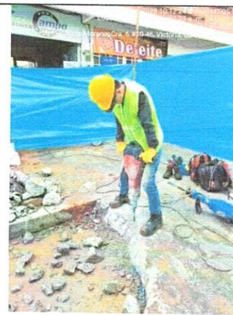
Ilustración 11: Demolición de placa existente
