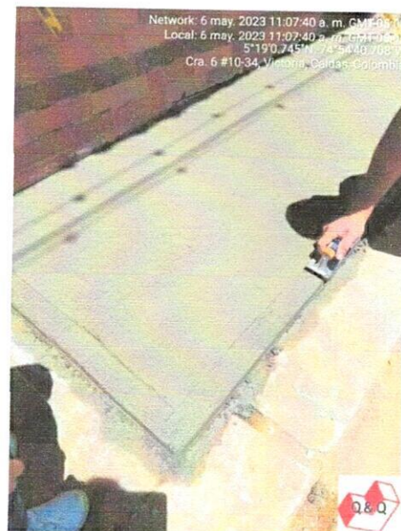
Ilustración 20: Vaciado y acabado de concreto para anden
