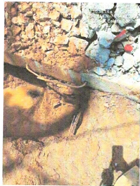
Ilustración 8: Domiciliarias existente en mal estado
