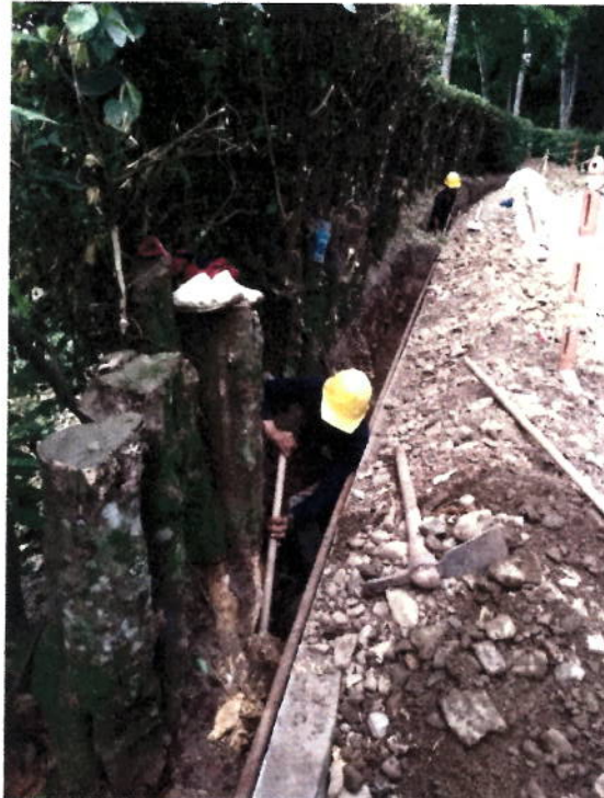
Excavación en Zanja
