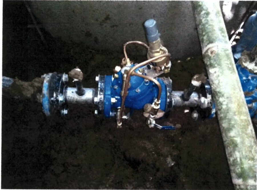
Instalación de válvula reductora de presión de 2"
