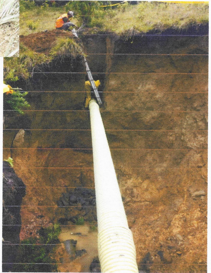
Fotografía No.11. Instalación de la tubería de 12".
