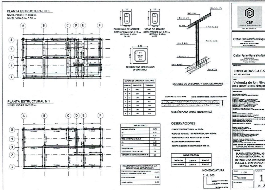
Ilustración 1 productos entregados por parte del contratista (planos de obra).
