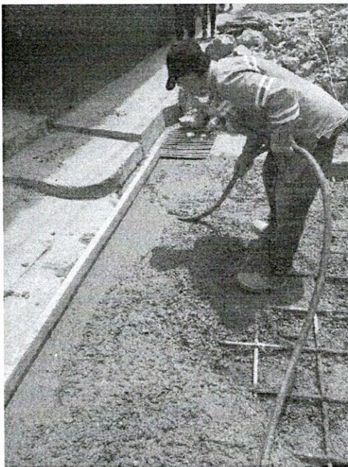
FOTO 7. Vaciado de concreto.
