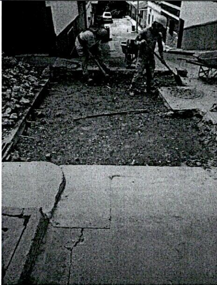
FOTO 1. Demolición del tramo a intervenir
