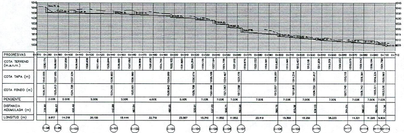
PERFIL COLECTOR 3
