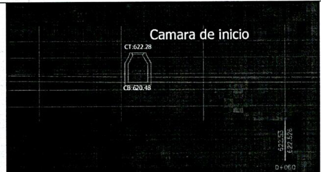
Cámara C2 (inicio del tramo a construir). Cota batea en CAD: 620.48 msnm. Cota Batea Calculada: 620.01 msnm
