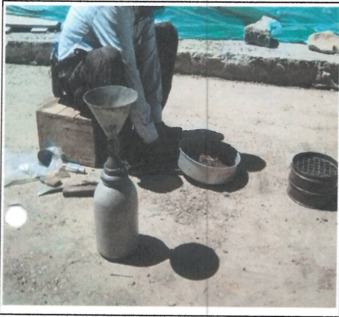
DENSIDADES SUBBASE GRANULAR PARQUE SAMANÁ
