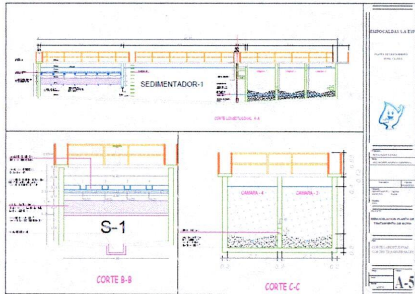
Actualización y levantamiento cortes generales de la planta tratamiento de agua del municipio de Supia, Caldas.
