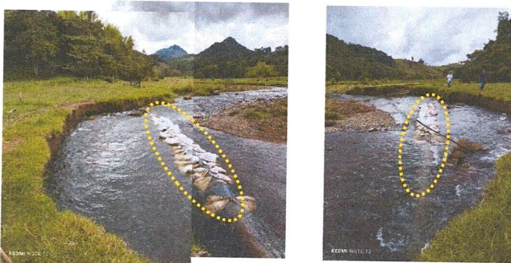
Fotos 7-8 (izquierda): vista hacia aguas arriba del punto crítico 3 y, foto 9: vista hacia aguas abajo. Procesos de erosión lateral más allá de la posición del tubo en este punto. Encerrado en óvalos, el tramo de tubería con presencia de costales rellenos de material aluvial para reducir la flotabilidad del tubo.
