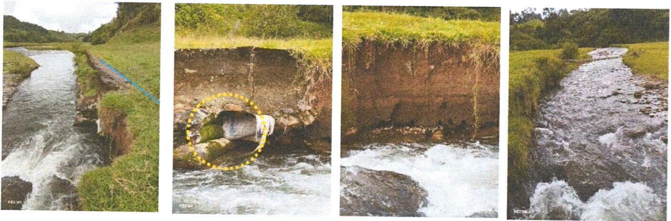
Fotos 1 a 4: Secuencia de imágenes que muestra, de derecha a izquierda, los procesos de socavación de orilla de aguas arriba hacia aguas abajo del punto 1
