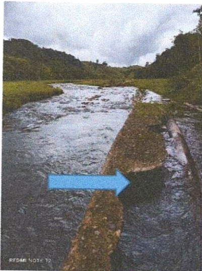
Fotos 5 (izquierda): vista hacia aguas abajo del punto crítico 2 y, foto 6: vista hacia aguas arriba. Procesos de erosión lateral y de fondo con compromiso total de la protección del tubo en este punto
