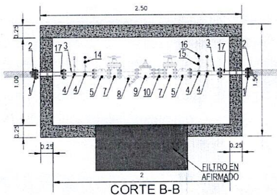
CORTE B-B
