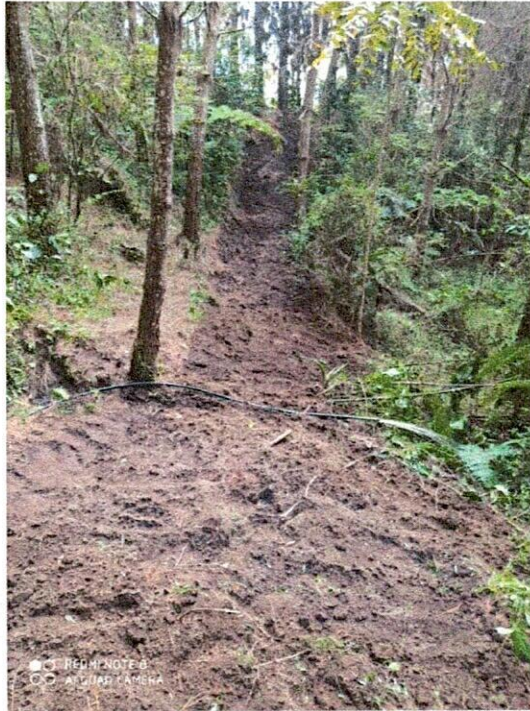
Imagen 23.- Rellenos compactos con material seleccionado de excavación posterior a instalación de tubería de polietileno de 10”.
