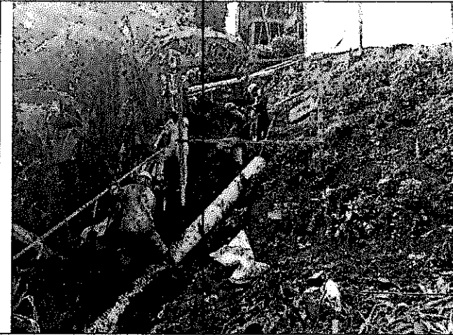
INSTALACIÓN DE TUBERÍAS
