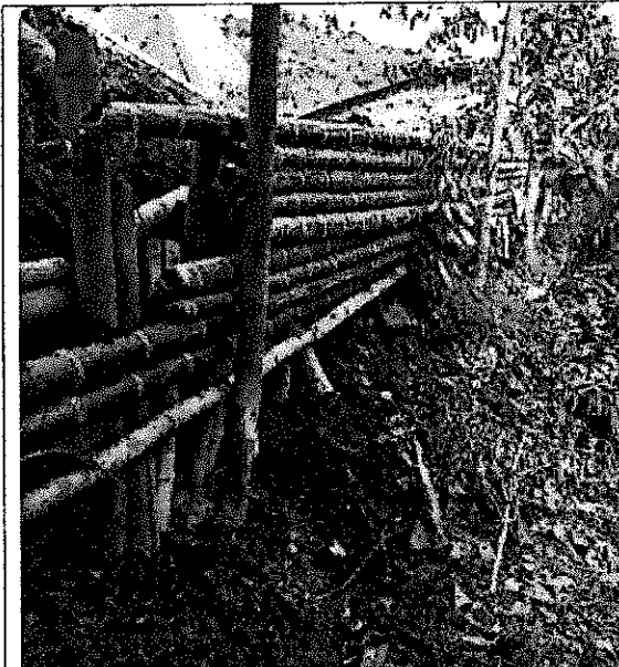
TRINCHOS PROVISIONALES PARA RETENCIÓN DE MATERIAL
