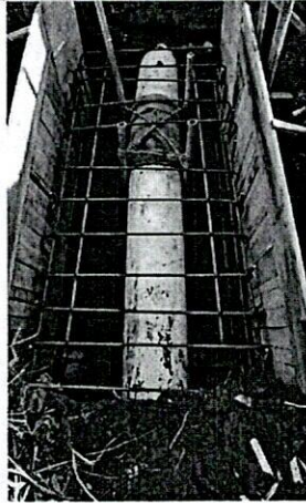
FOTO 3. Armado de hierro para fundición del anclaje
