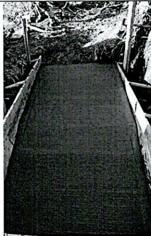
FOTO 3. Armado de hierro para fundición del anclaje
