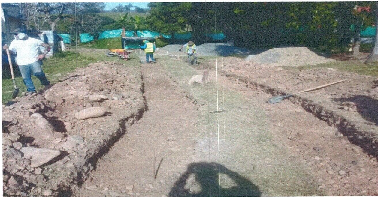
NIVELACIÓN DEL TERRENO POR LAS CINTAS EN CONCRETO
