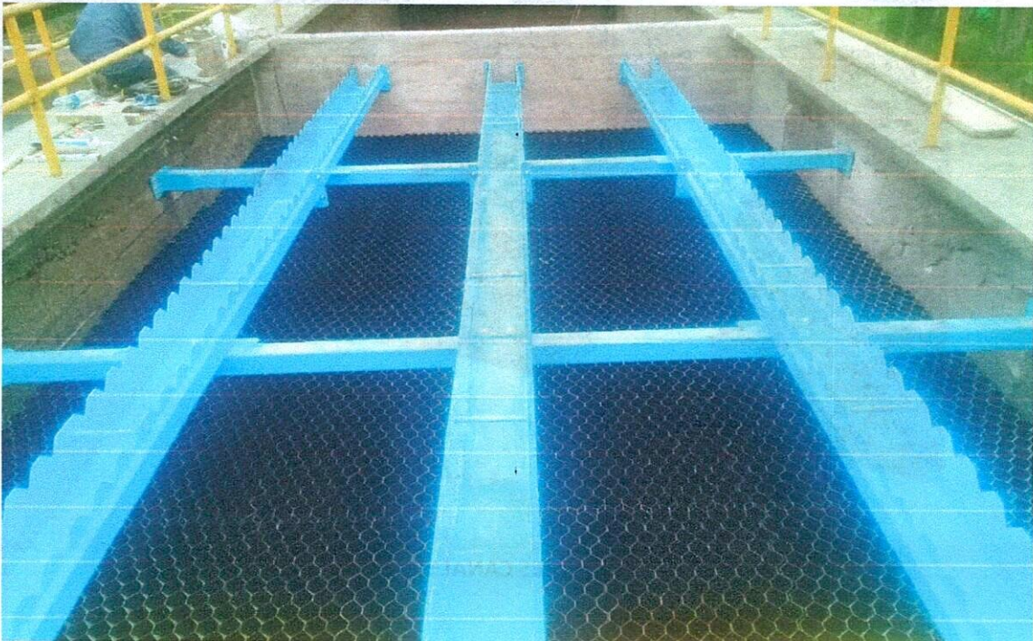
CANALETA DE RECOLECCIÓN Y MÓDULO DE SEDIMENTADOR 2
