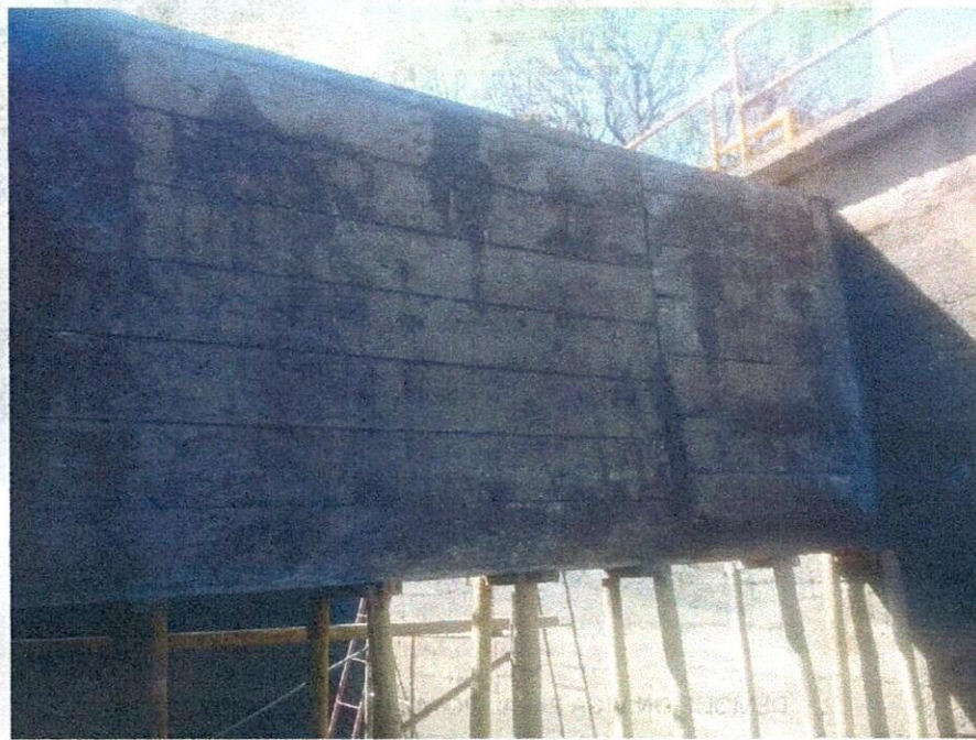
PANTALLA NUEVA EN FLOCULADOR 2
