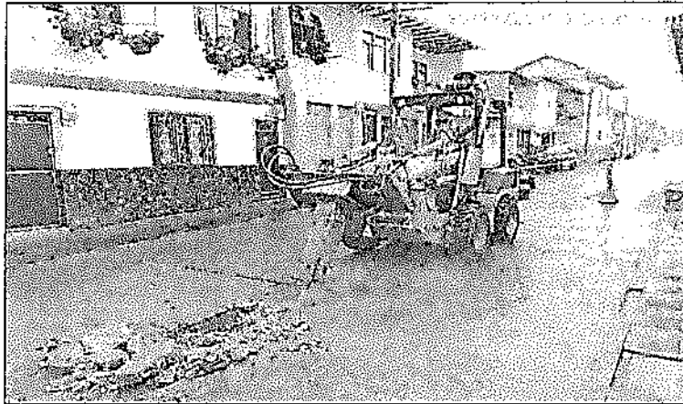
(demolición de zanja para tubería de 12")
