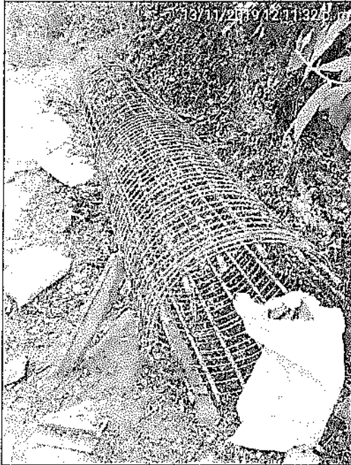
(canastillas de refuerzo y anillado para los caisson)
