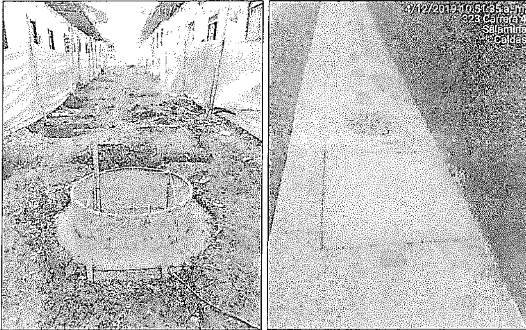
(cámara de caída y cajas de inspección sobre andenes)
