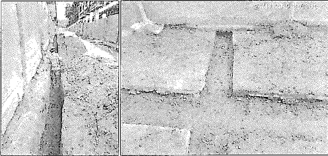
(excavaciones para red madre y acometidas domiciliarias)
