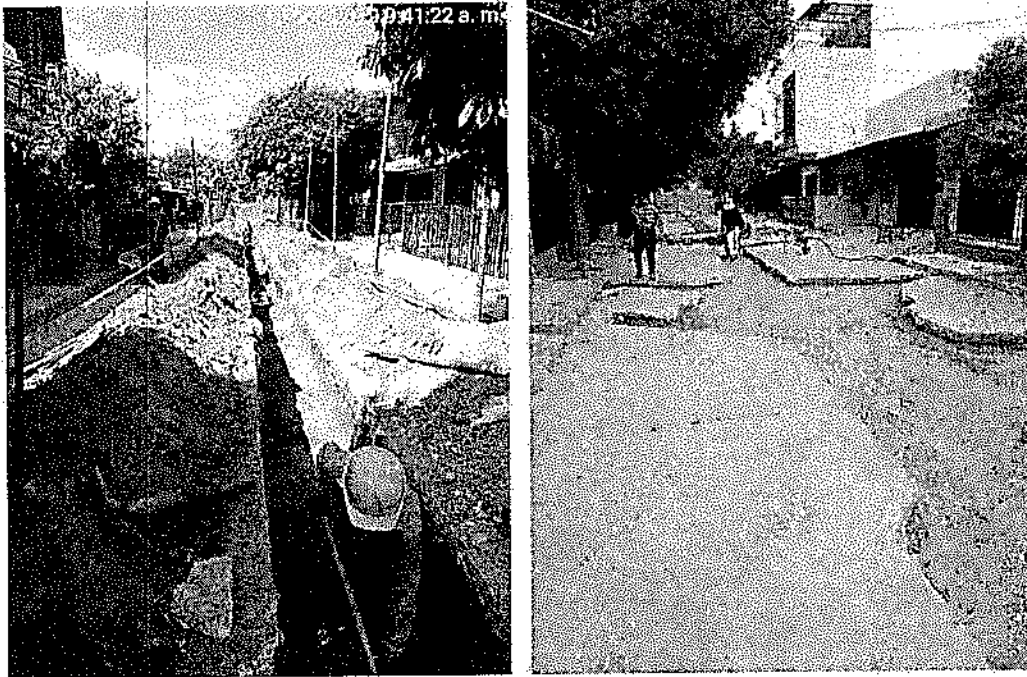
Fotografías 5 y 6: Se ejecutó la obra con normalidad, la estructura del pavimento sufrió un asentamiento por mala compactación, lo que generó grietas en el concreto hidráulico.
