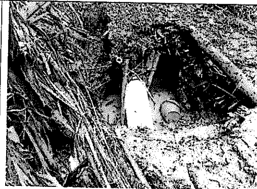
Reparación mediante la instalación de 12 metros de tubería de polietileno
