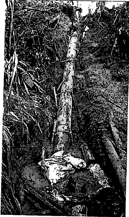
Reparación mediante la instalación de 12 metros de tubería de polietileno instalación de anclajes en concreto y tubería galvanizada
