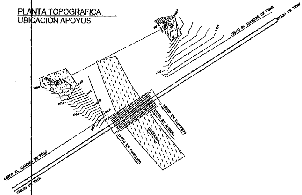
Levantamiento zona denominada sector km 41.
