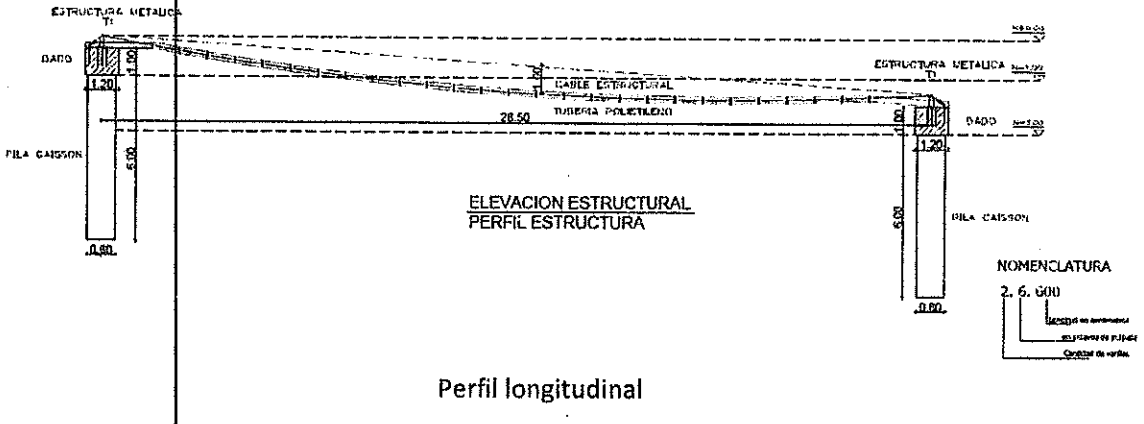
Piano diseño viaducto sector Arauca.
