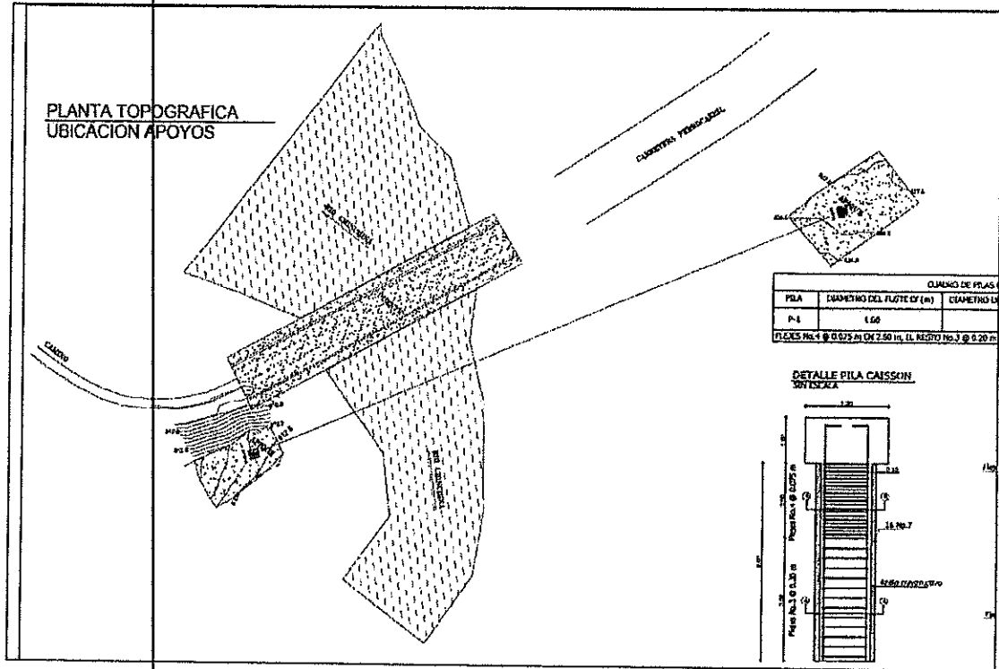
Levantamiento topografico zona denominada sector Arauca.
