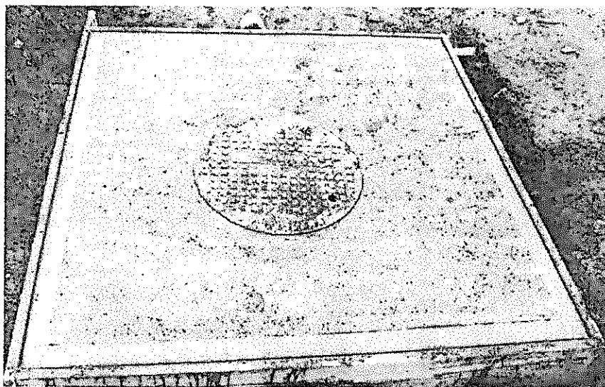
INSTALACION DE LOSA CON TAPAS PARA POZOS DE INSPECCION
