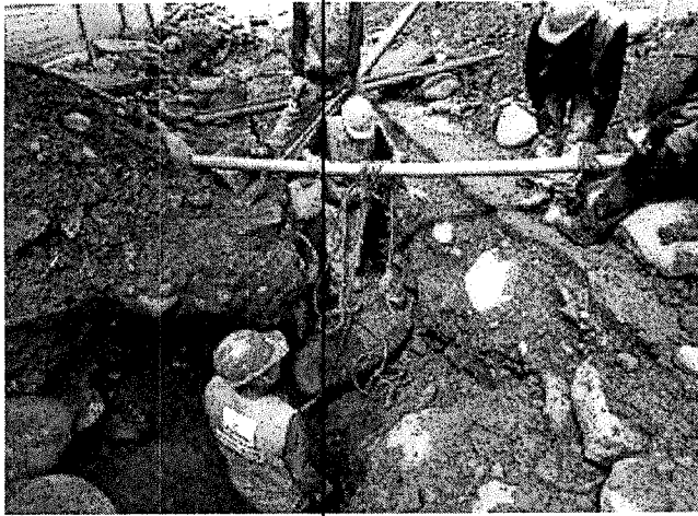
RETIRO DE ROCAS DE GRAN TAMAÑO MEDIANE LA UTILIZACIÓN DE ZOGAS Y TELERAS
