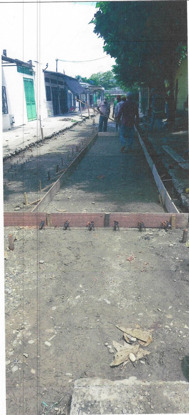
Imagen 1. Instalación de formaleta para losas.
