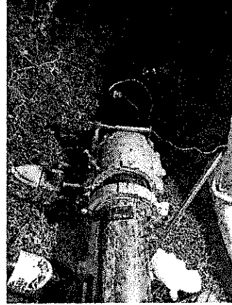
INSTALACIÓN DE TUBERÍA D EPOLIETILENO DE 6" 84 METROS
