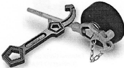
Llaves para operación y reparación de hidrantes
