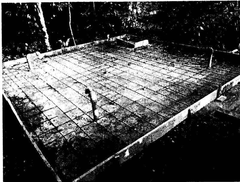
Reforzamiento tapa de tanque.
